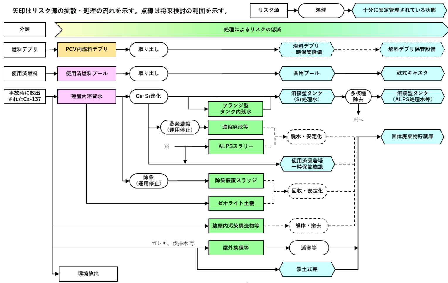
(a) リスク低減プロセス
