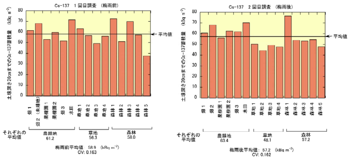
図 21. 表層の植生・リターを含む深さ 20cm までの放射性セシウムの蓄積量（本図はセシウム 137 の例）（平均値は算術平均）
