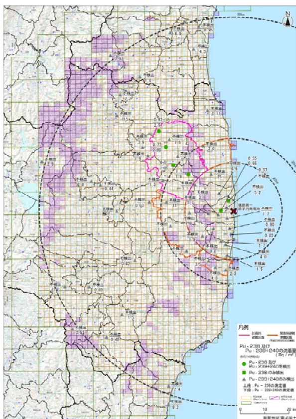
図 12. プルトニウム 238、239+240 の 土壌濃度マップ（平成 23 年 6 月 14 日 時点に放射能濃度を換算）
