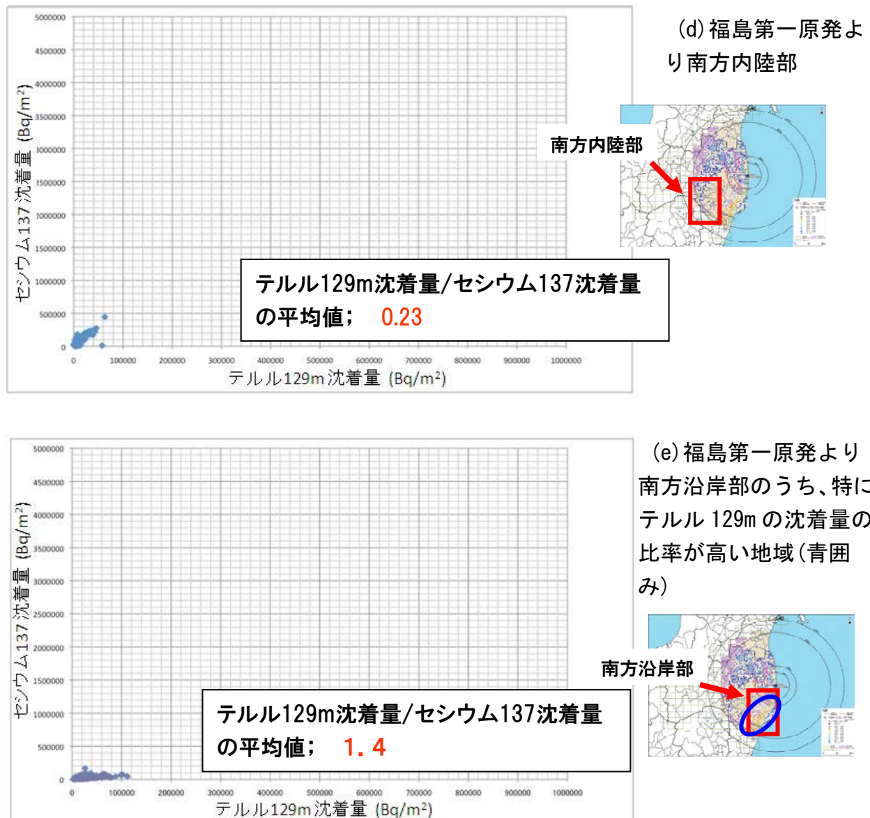
図 11. セシウム 137 とテルル 129m の沈着量の相関関係 (その 2)
