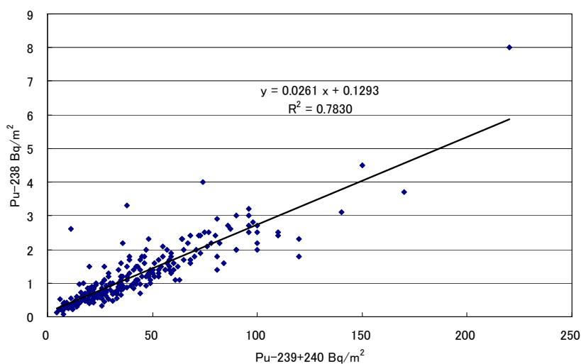
図 14. 平成 11～21 年度までの環境放射能水準調査の結果（プルトニウム 238 とプルトニウム 239+240 の沈着量の関係）（平成 11 年～21 年までに採取された土壌 1,054 試料のうち、プルトニウム 238、プルトニウム 239+240 が検出された 252 試料の測定結果を比較）
