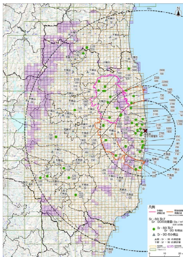
図 13. ストロンチウム 89、ストロンチ ウム 90 の土壌濃度マップ（平成 23 年 6 月 14 日時点に放射能濃度を換算）
