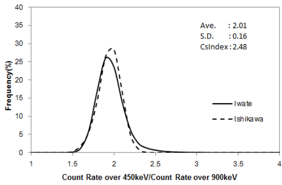
Fig. A3-18 OYO; Histogram of Cs-index
