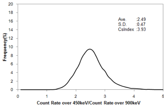
Fig. A3-20 Histogram of Cs-index in Kyusyu 1
