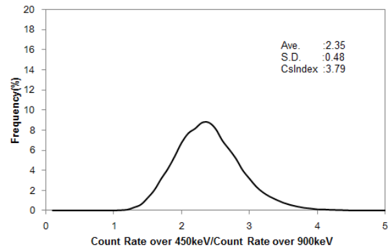
Fig. A3-21 Histogram of Cs-index in Kyusyu 2
