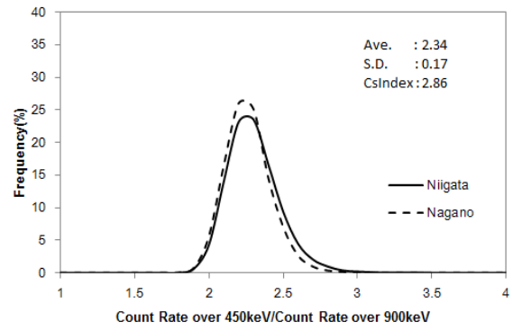
Fig. A3-17 NUSTEC; Histogram of Cs-index
