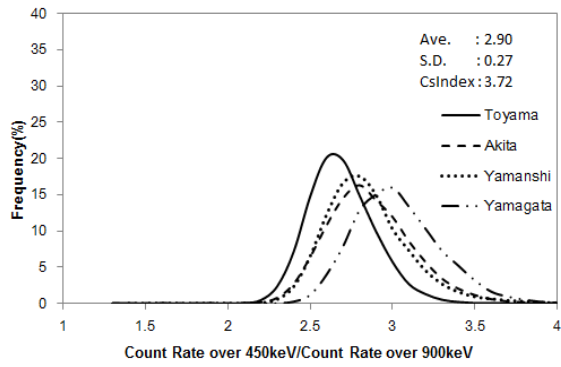
Fig. A3-16 MEXT-1; Histogram of Cs-index
