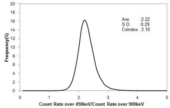
Fig. A3-25 Histogram of Cs-index in Kinki 2
