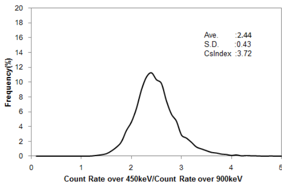
Fig. A3-22 Histogram of Cs-index in Kyusyu 3
